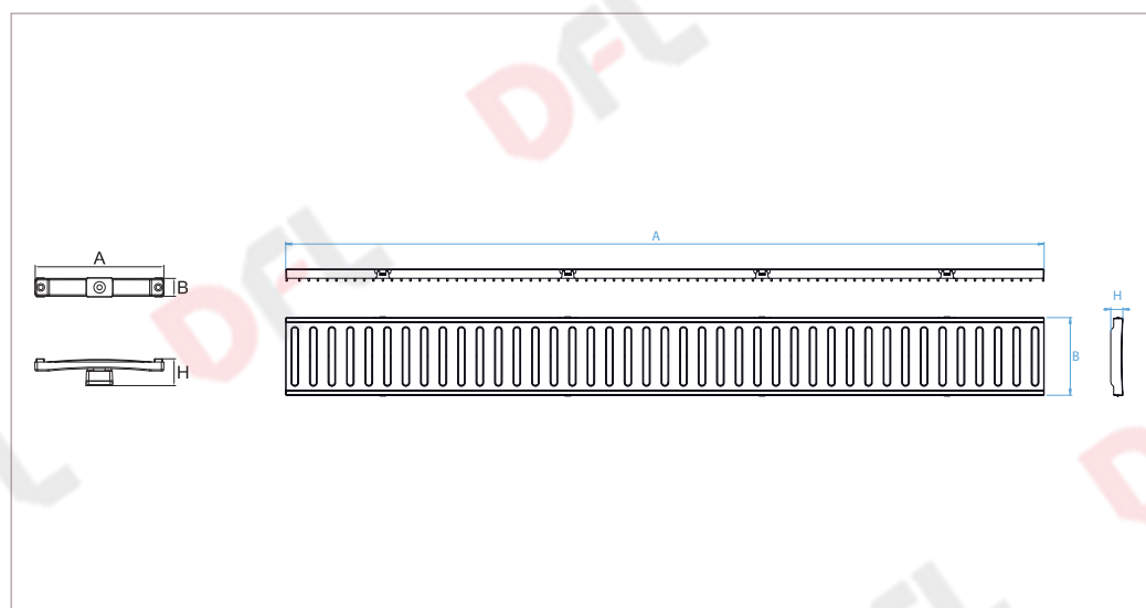
Sistema autobloccante della griglia
